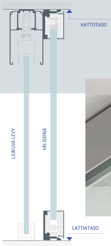
■ Leikkaus 3-3
