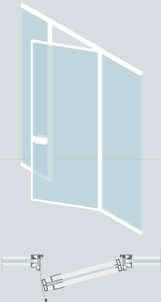
1. Levy profilissa ALU 1 / Kääntö
