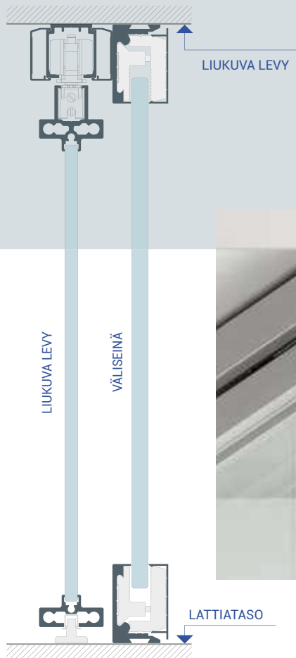
■ Leikkaus 1-1
