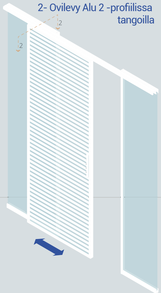
■ Leikkaus 2-2
